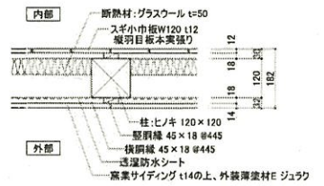
基本外壁 凡例 S:1/10 ※ 間柱:40x120 #445
