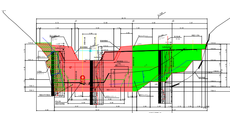
堰堤正面図
