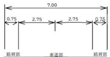
標準断面図（改良後）
