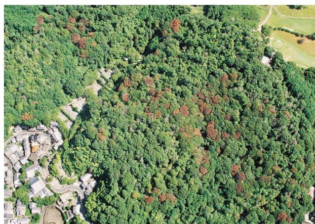
ナラ枯れの発生状況(2009年8月)
