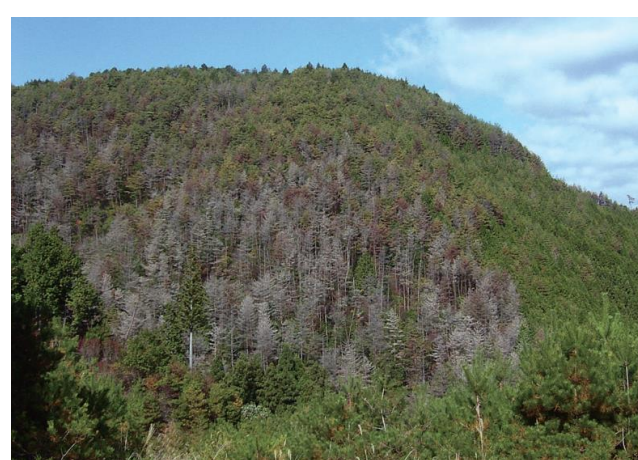
マツ枯れの発生状況(2007年11月)
